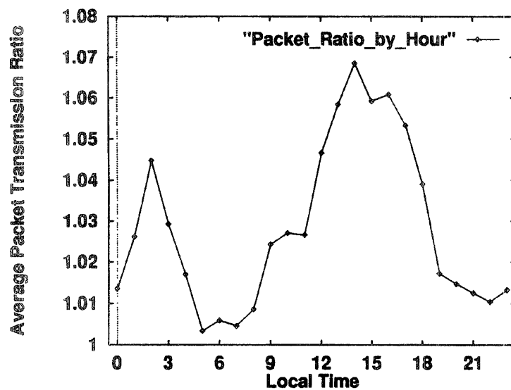
第4図. 時間毎の平均実パケット比
