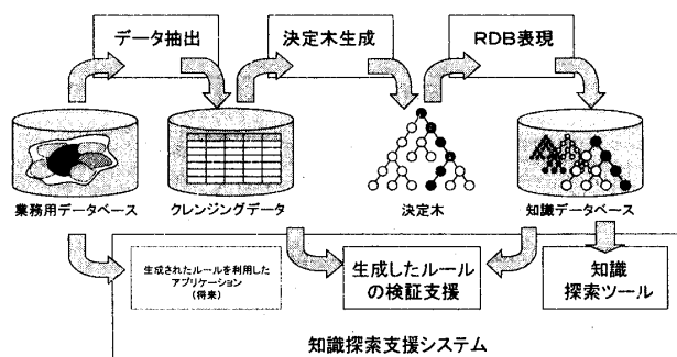
図1 本研究の概要
